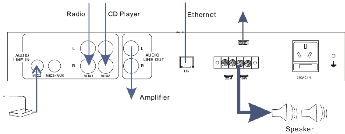
Рис.3.1. Схема подключения LPA-8508NASP06
